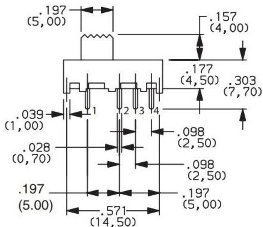
Actuator shown in pos. 1
